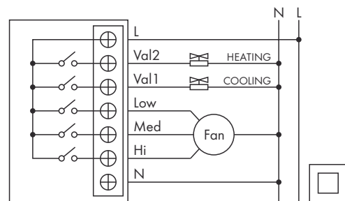
SCHEMAT POŁĄCZEŃ / WIRING DIAGRAM
