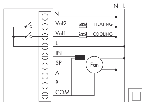
SCHEMAT POŁĄCZEŃ / WIRING DIAGRAM
